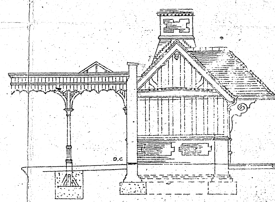
End Elevation F.F.
