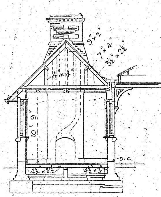
Section D.D.
